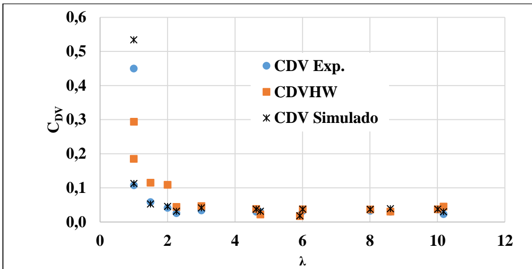
Figura 9: Gráfico dos coeficientes de arrasto experimental, analítico e simulado
